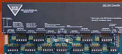
Module Ex-1044 32 entrées alarme 4 sorties relais
